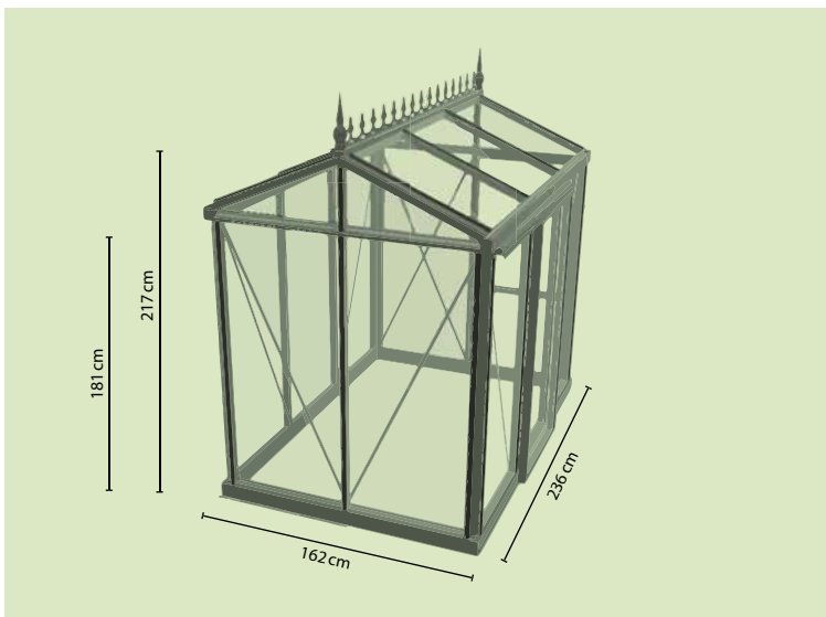
Gewächshaus Helios Urban
